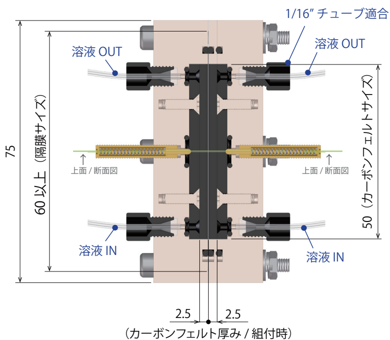
セル 正面 / 断面図 ●
