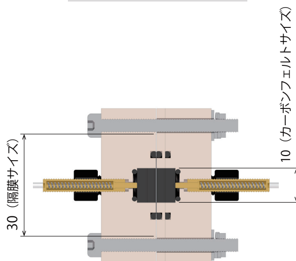
セル 上面 / 断面図 ●
