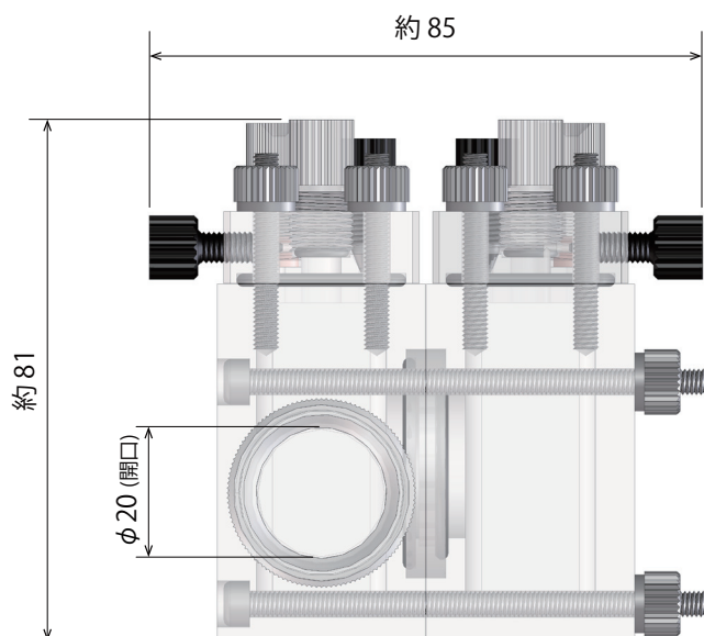
セル 正面図
