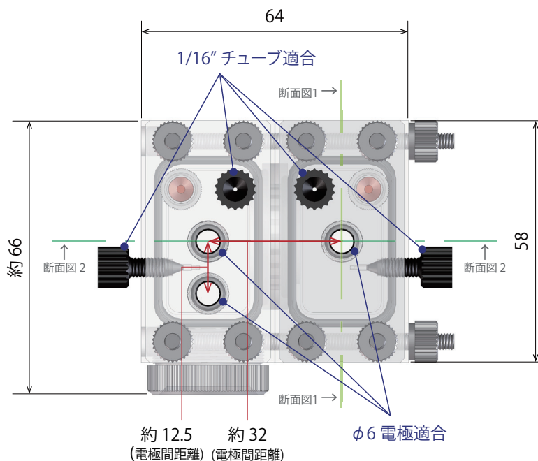
セル 上面図
