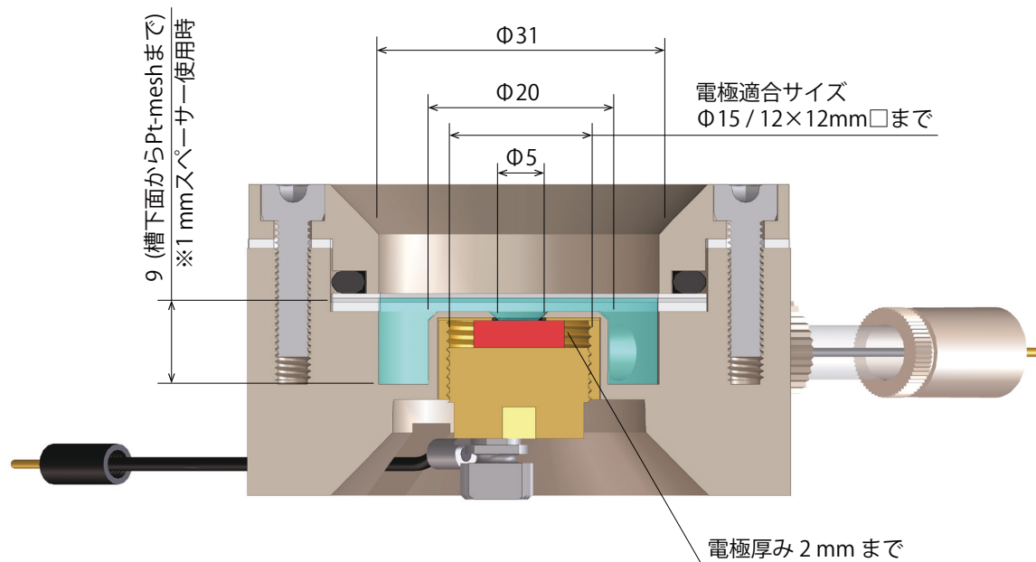
〈電解槽部寸法図〉
