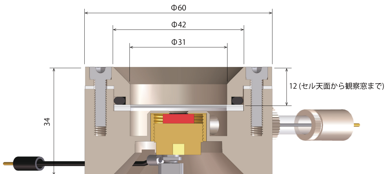
〈対物レンズ対応寸法図〉
