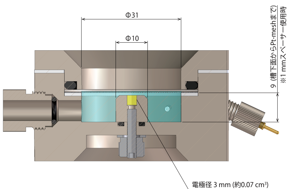
〈電解槽部寸法図〉
