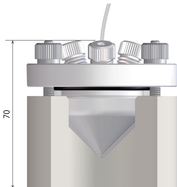
セル正面図
