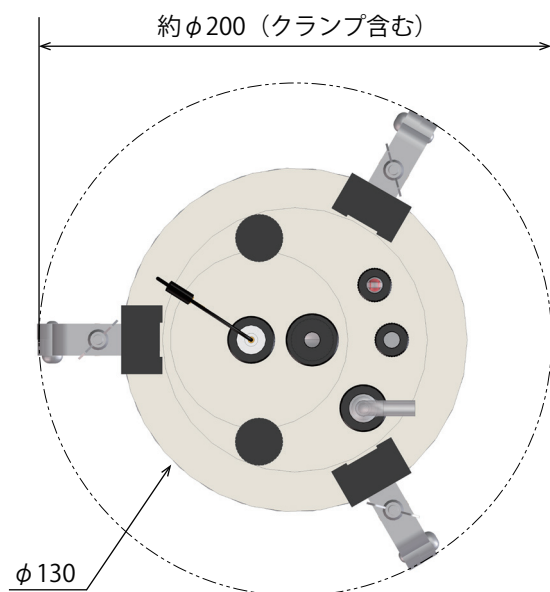
セル 上面図
