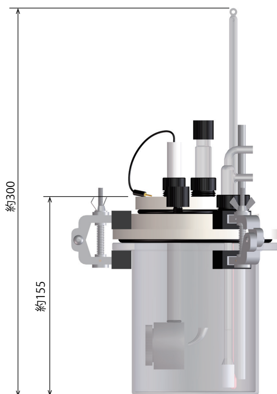
セル 正面図
